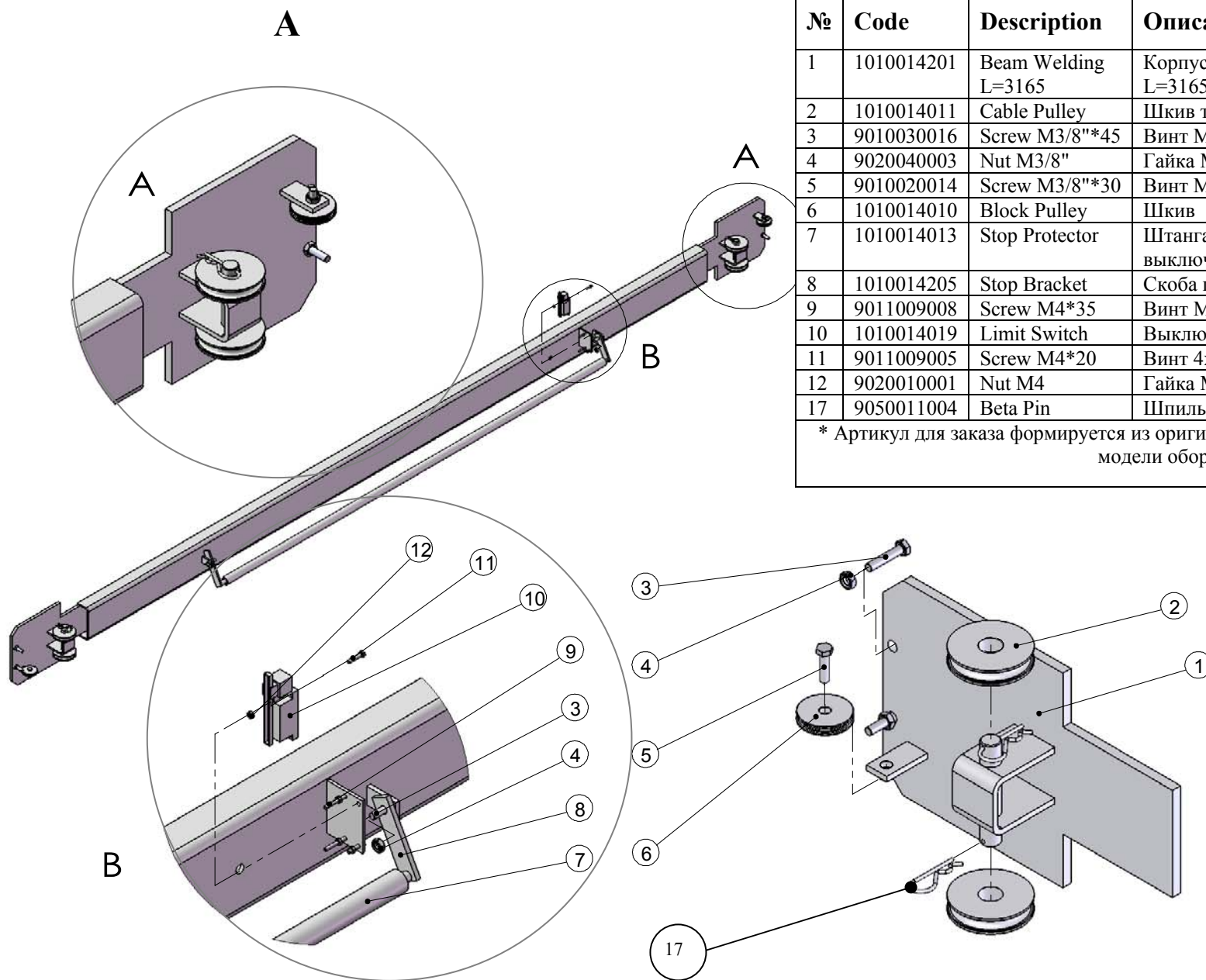
Переключатель в сборе (1010014100)
