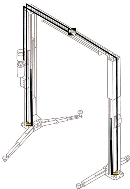
Схема прокладки гидравлических шлангов
