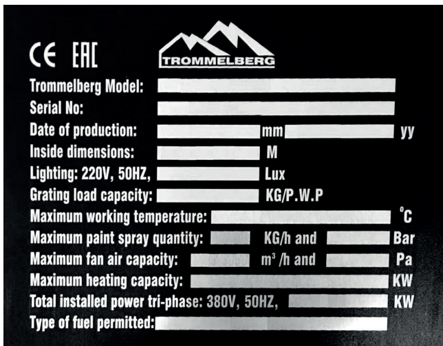
Рис. 5 Идентификационная табличка на агрегате Расшифровка идентификационной таблички
